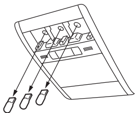
② 電球の取外し
